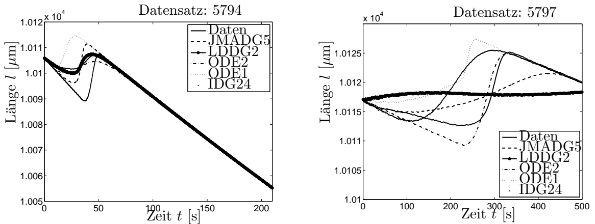
Abbildung 6: Zurückgerechnete Längen der nicht–isothermen austenisch–perlitischen Umwandlung bei linearer Abkühlung
