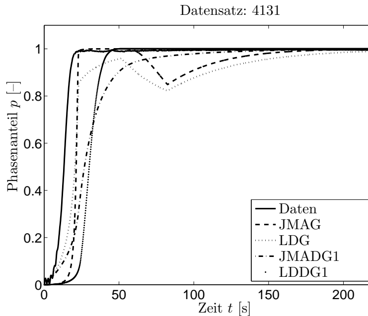
Abbildung 1: Unterschiede zwischen den algebraischen Gleichungen und den Differentialgleichungen von Johnson–Mehl–Avrami und Leblond–Devaux
