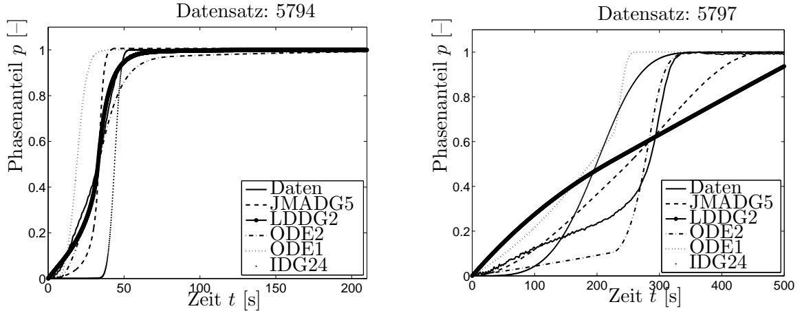
Abbildung 5: Phasenanteile der nicht–isothermen austenisch–perlitischen Umwandlung bei linearer Abkühlung
